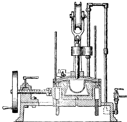
Hat-Mold.
