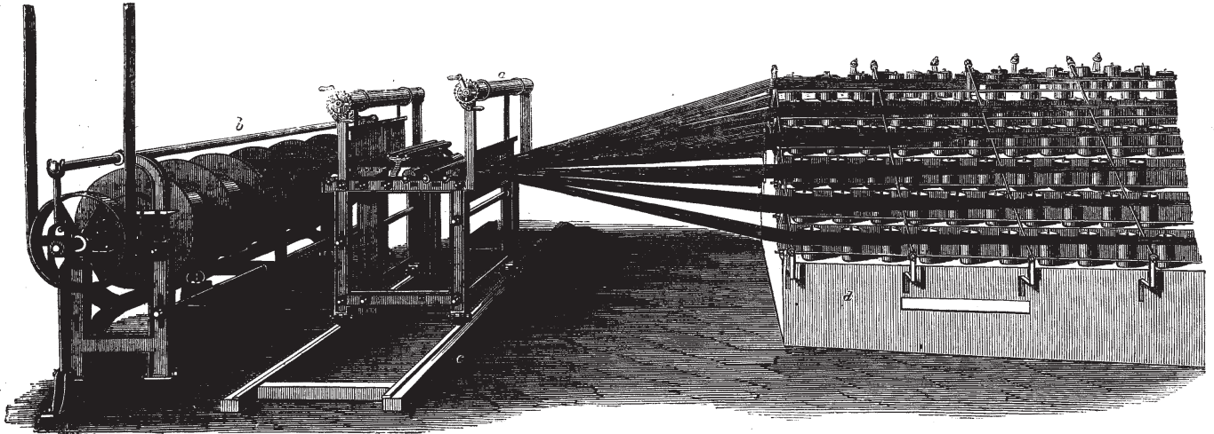
WARPING FRAME, CONSTRUCTED BY THE ERSTE BRÜNNER MASCHINEN-FABRIKS GESELLSCHAFT BRÜNN.
