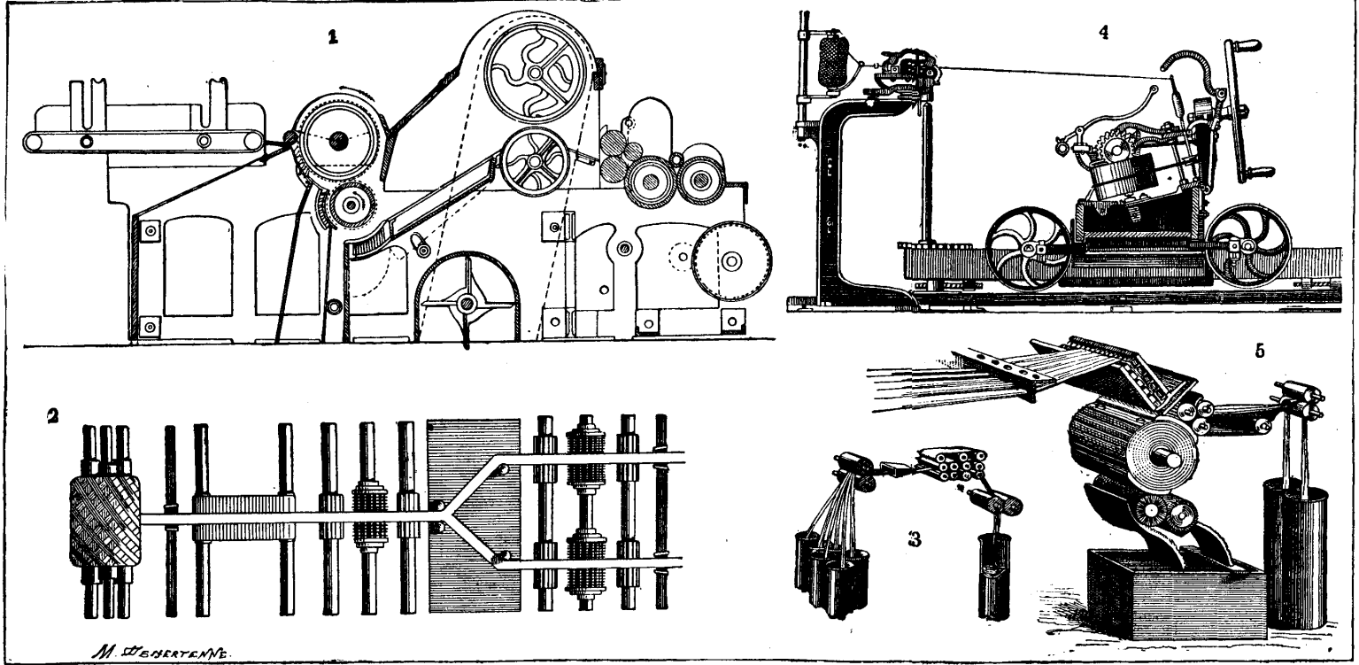
Filature : 1. Carde ; 2. Défuteur étireur ; 3. Doubleuse étireuse ; 4. Mull Jenny ; 5. Peigneuse.
