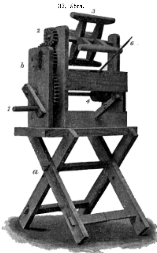
Japáni selyemgombolyító-gép távlati előrész. A természetes nagyság \frac{1}{10} -de.
