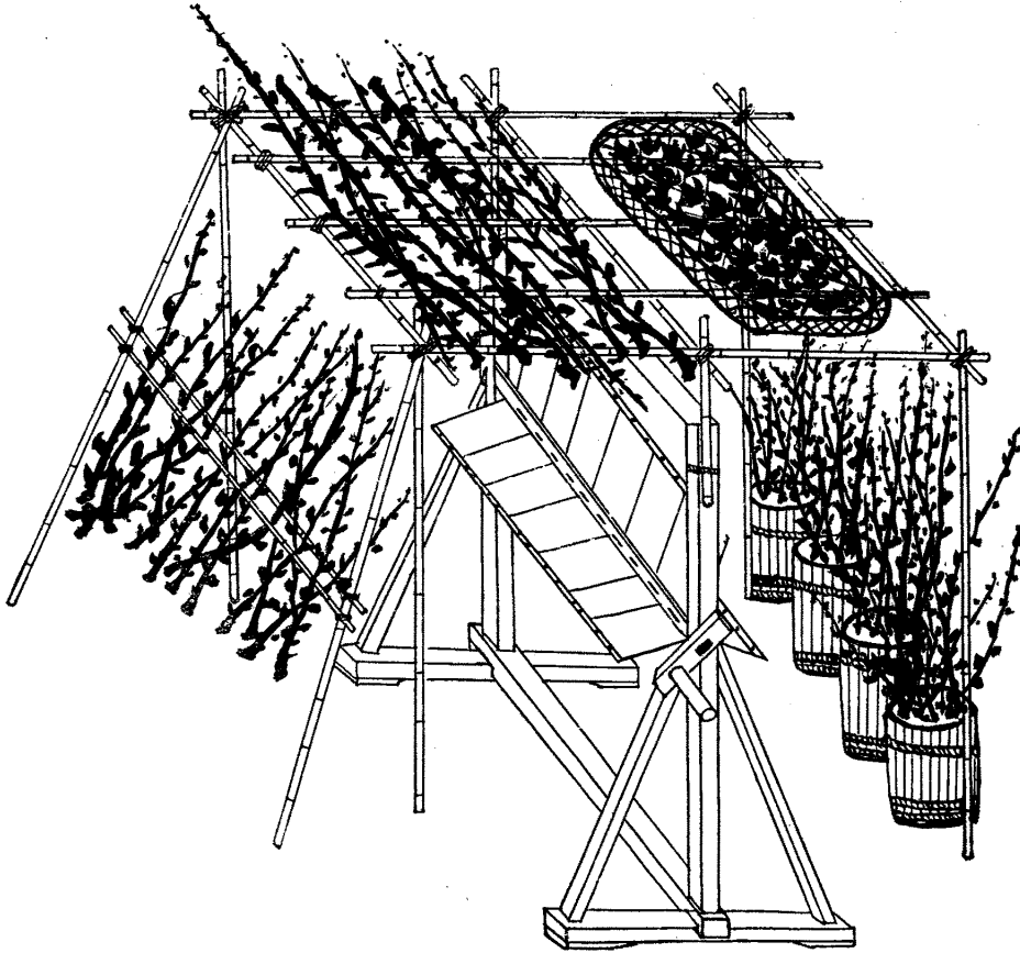
A lombzárításra szolgáló szélmalom. 1 : 25.
