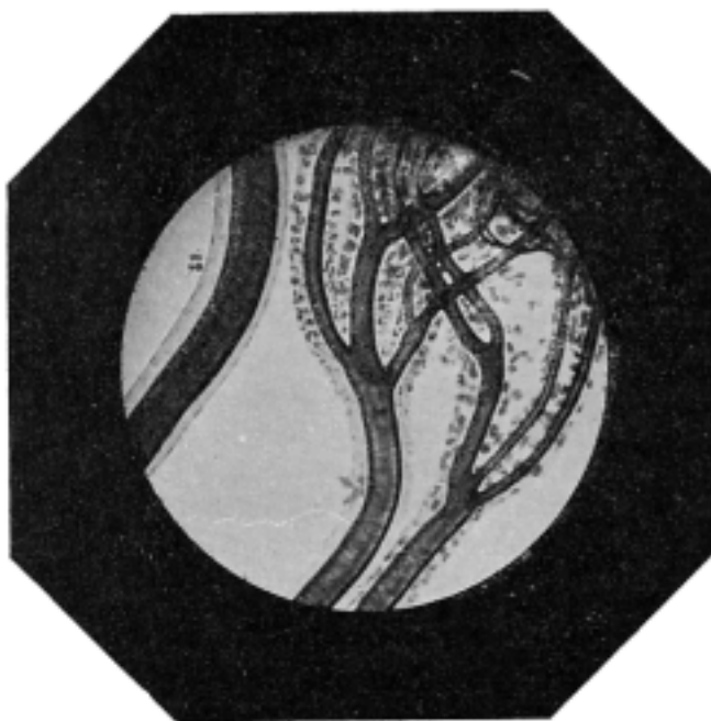
Egy trachea mikrophotographiája, melynek peritracheal-szöveve polyeder-szemcséket tartalmazó cystát visel. Balra egy egészséges trachea. 200-szor nagyítva.
