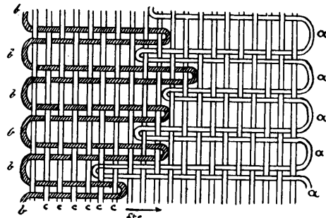
Fig. 209
