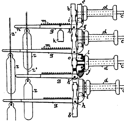
Fig. 241
