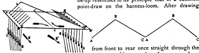
FIG. XXXV.
