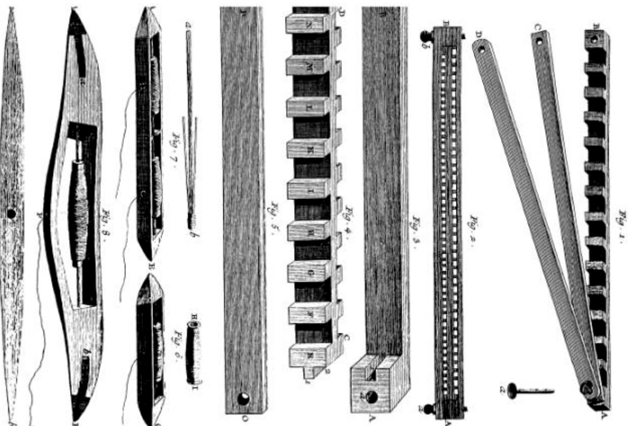
Soierie, Escalier, Trepelous, Vantelle 8c.
