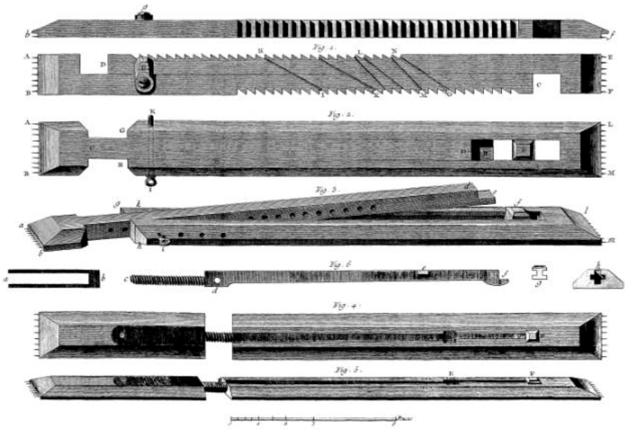
Soierie, Tempia de differantas sortes, Tempia à Corde, Tempia à Bouton et Tempia à Vis.
