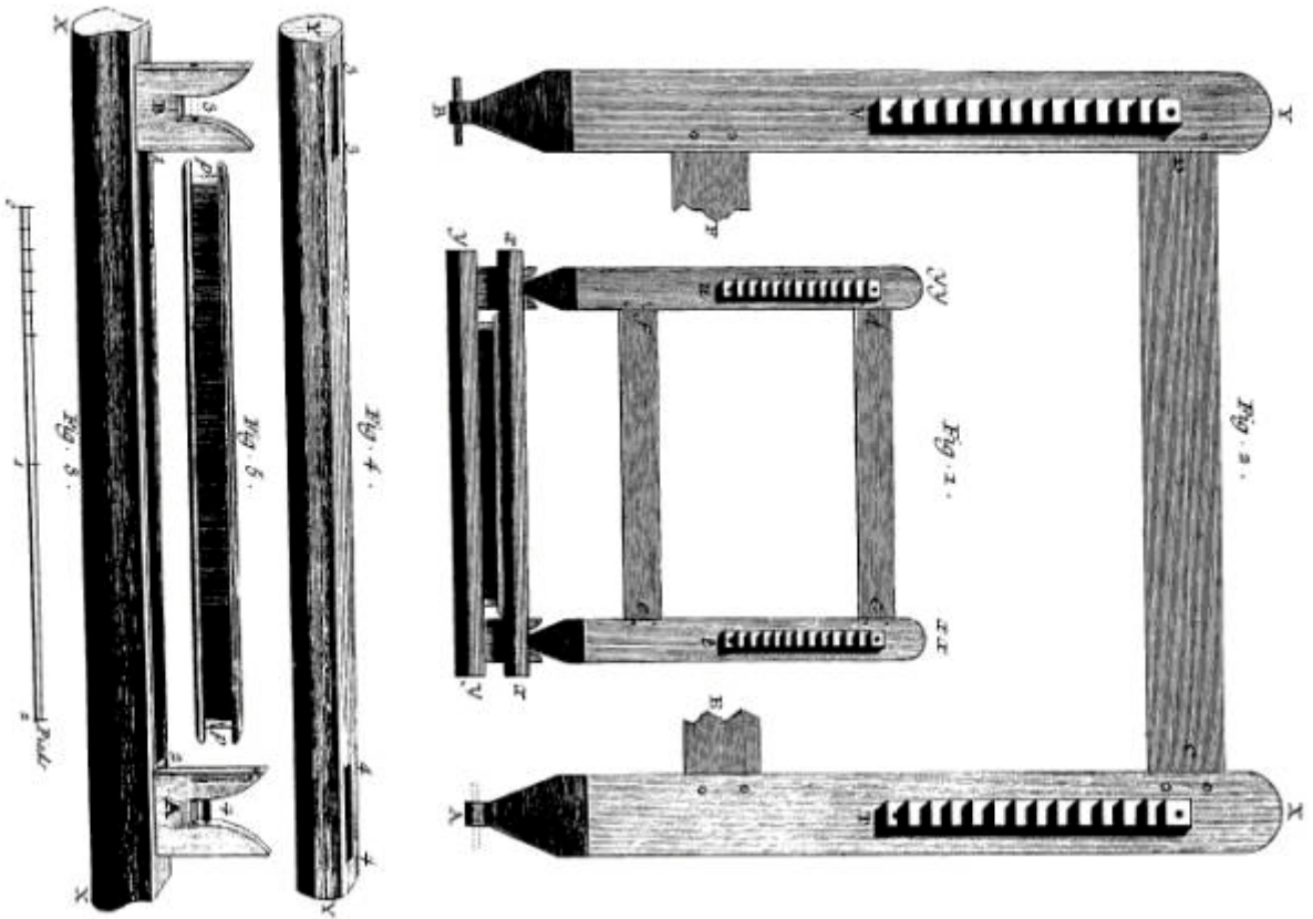
Soierie. Velours. Développement du Râteau brisé du Mouton à Velours.
