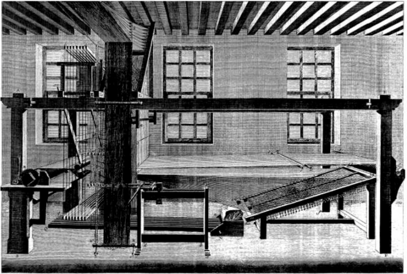
Soierie, Vélours. Élévation Perspective du Métier pour fabriquer le Vélours Ciséle, vu dans l'instant de la Tire et du Pédage des Fers.
