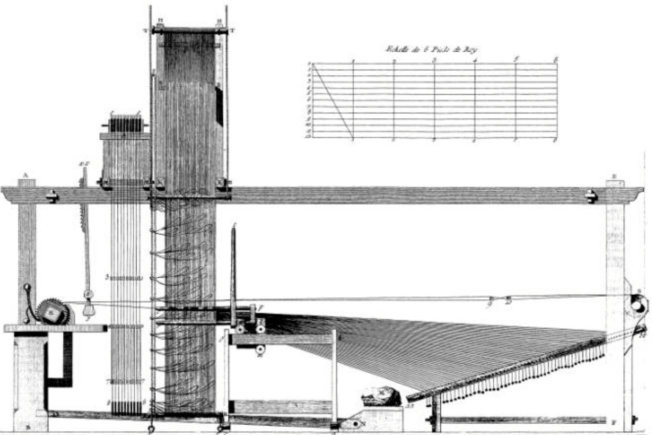
Soierie, Vélours. Élévation Latérale du Métier pour fabriquer le Vélours Ciséle Vu dans l'instant qui précède celui de la Tire.
