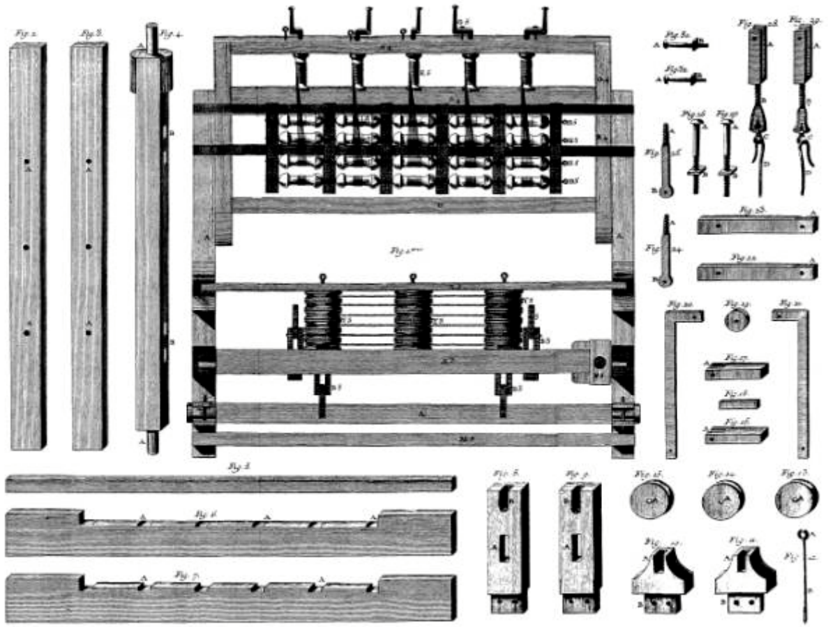
Métier à faire le Ruban. Plan du défilé.
