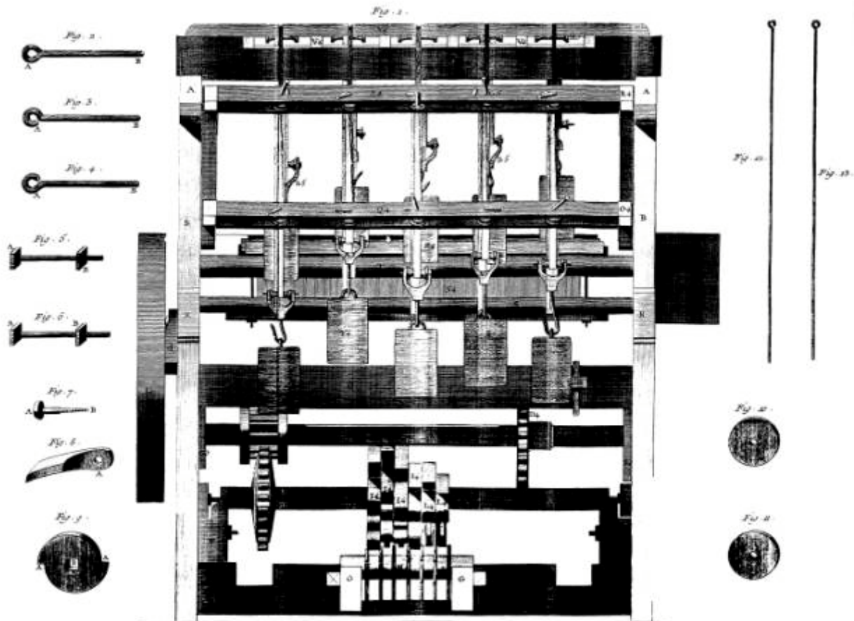
Métier à faire le Ruban, élévation par derrière.
