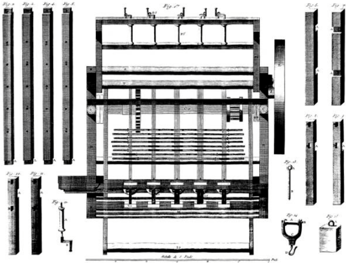
Métier à Ruban, Plan des Lames.
