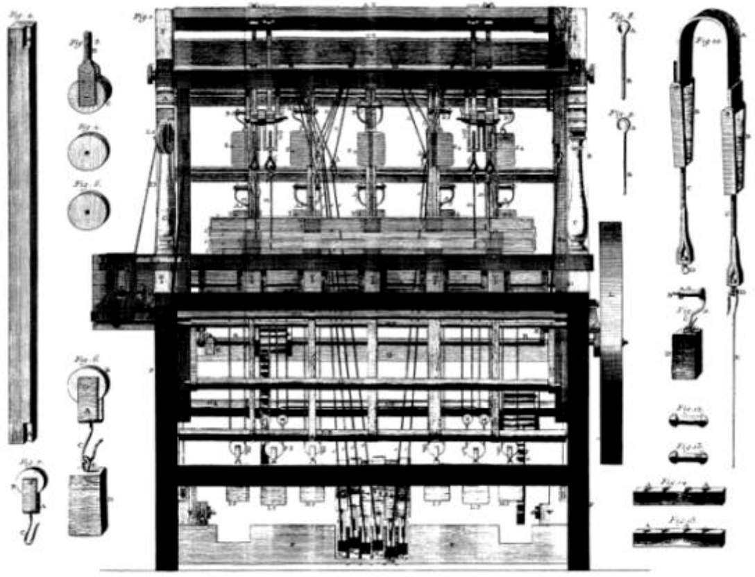
Métier à faire le Ruban, Élévation en face.
