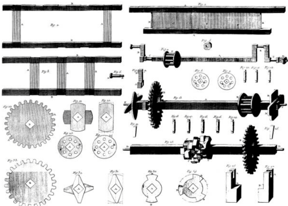
Métier à faire le Ruban, Développement
