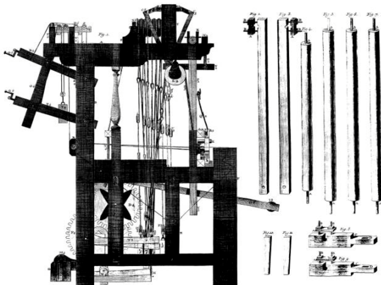
Métier à faire le Ruban, élévation latérale.
