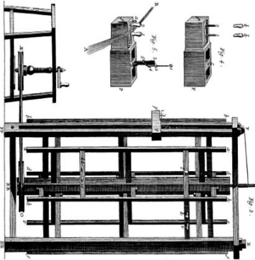
Soierie, Développement de l'ourdisoir.
