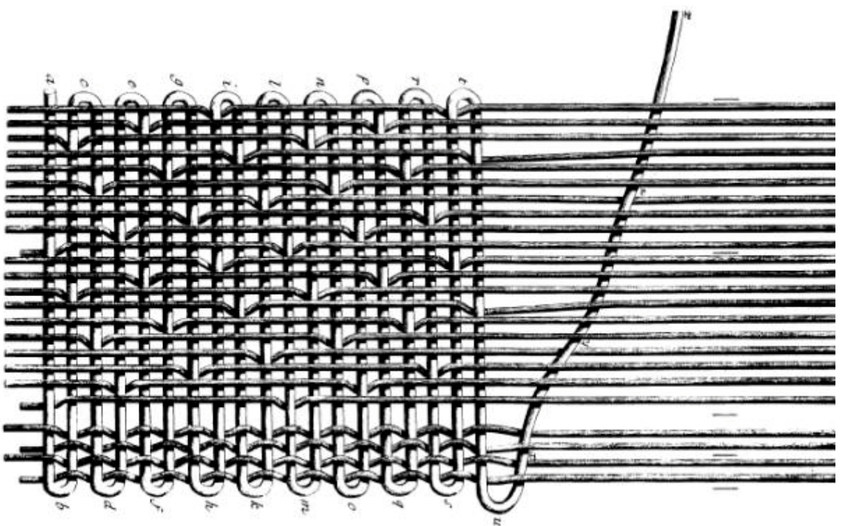
Soierie, Broyée en Plein, selon à deux Traverses Par du côté de l'ouvrier.
