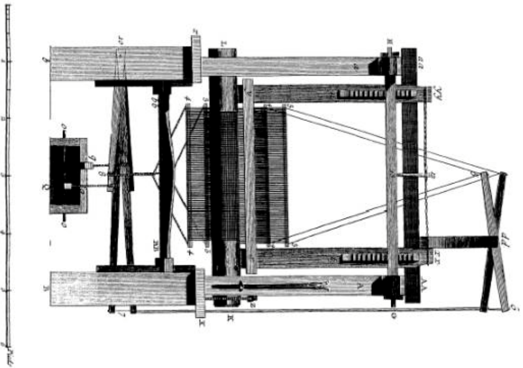
Soierie, Elevation Generale de la partie anterieure du Meier pour fabriquer les Rieffes sans, comme Tuffin, Sibir, et soye
