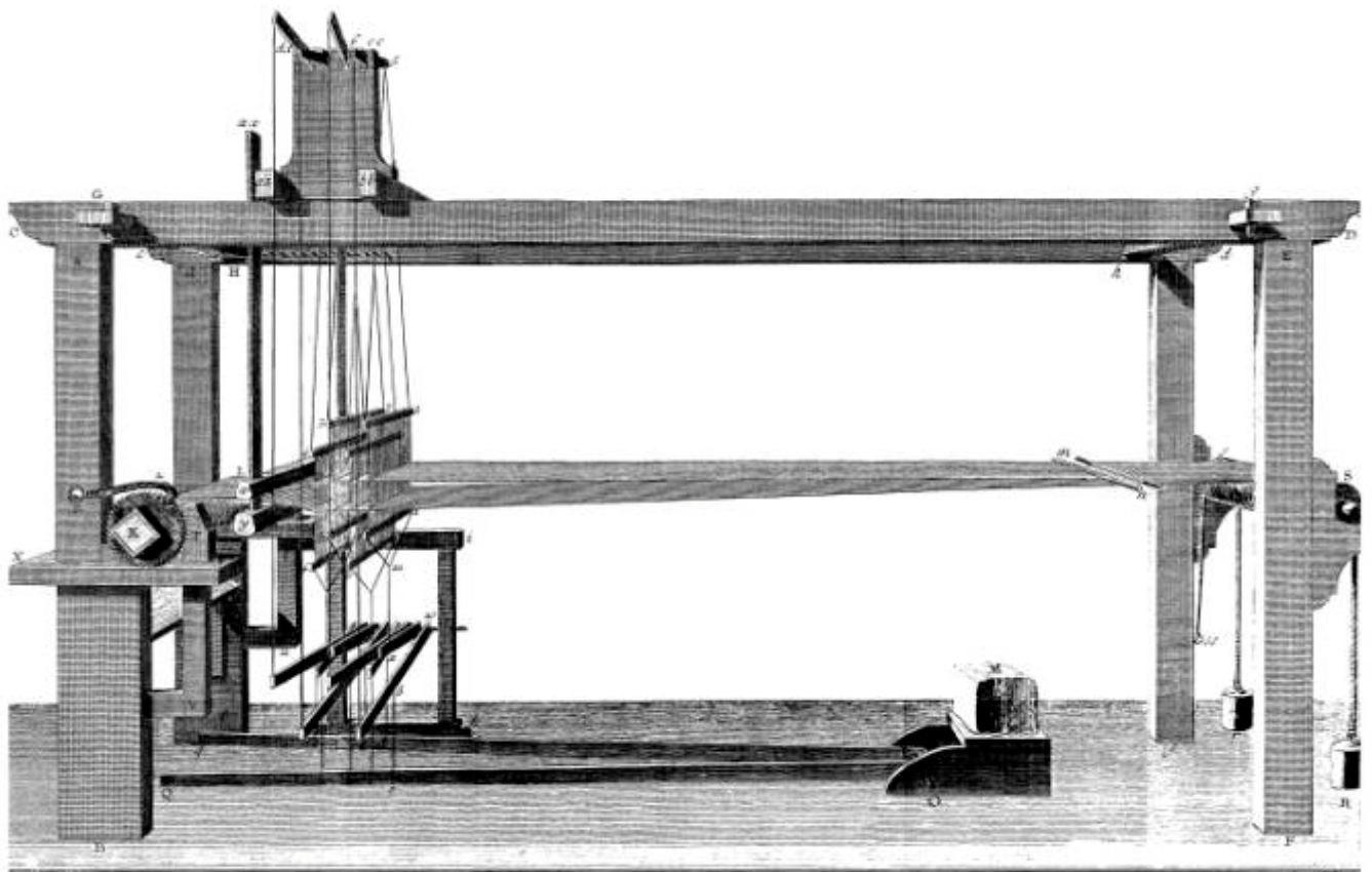
Soierie, Vue Perspective du métier pour fabriquer les Étoffes unies, comme Tafetas, Satin et Serge, la Chaîne ouverte au premier coup du Tafetas H
