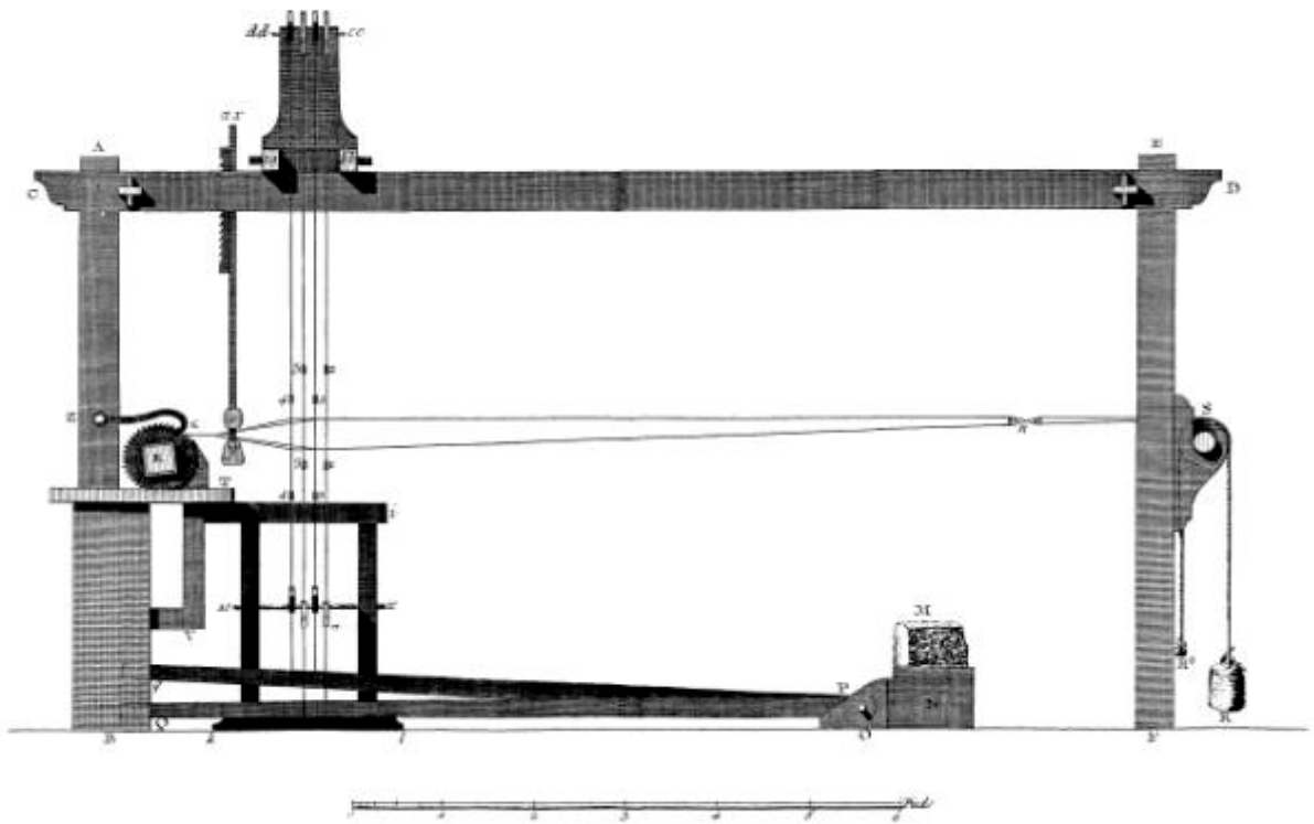
Soierie, Elevation Géométrale de la partie Laterale du métier pour fabriquer les Étoffes unies, comme Tafetas, Satin et Serge
