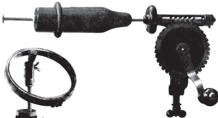
Nr. 5056 Spoleapparat til at spole Traaden paa Kniplepinde. Spolen kan gaa mellem 3-4000 Omdrejninger pr. Minut. Kr. 5.- 10/-
