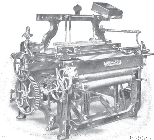
Plain Calico Loom
